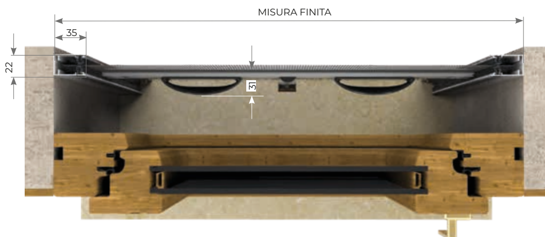
VARIANTE A RICHIESTA AGGANCIO PIATTO
