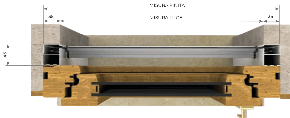
AGGANCIO MAGNETICO
