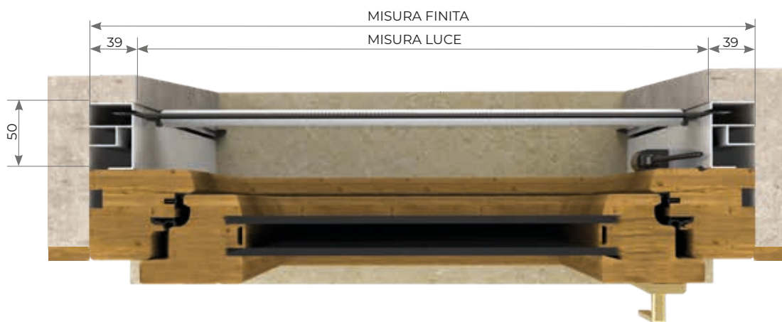
OPTIONAL AGGANCIO MAGNETICO
