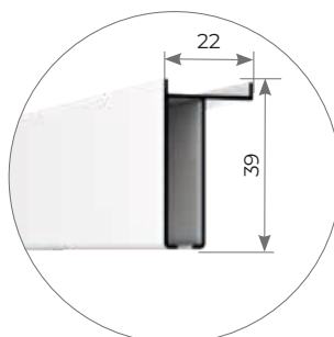
GUIDA SUPERIORE STANDARD
